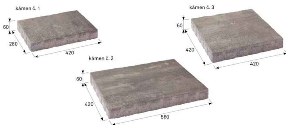
Skladebné rozměry, sestava 3 druhů kamenů
